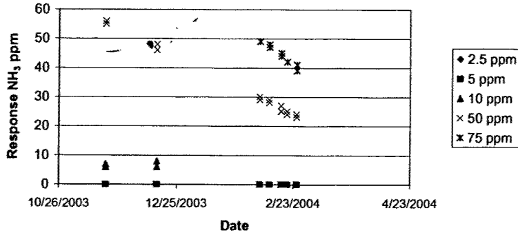
Figure 13. iTX NH 3 Sensor
