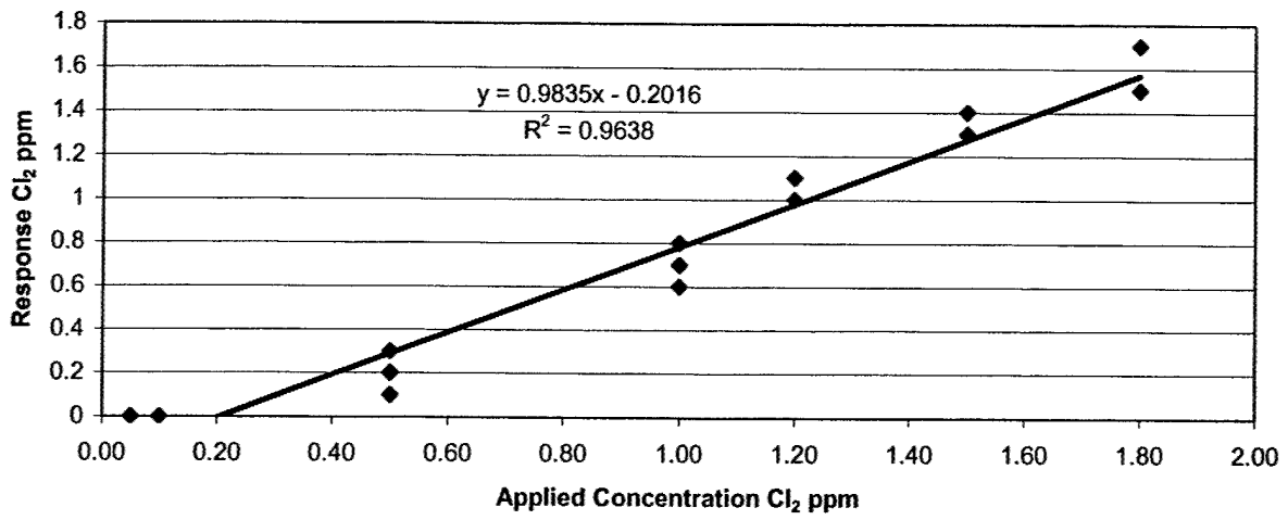
Omni Cl 2
