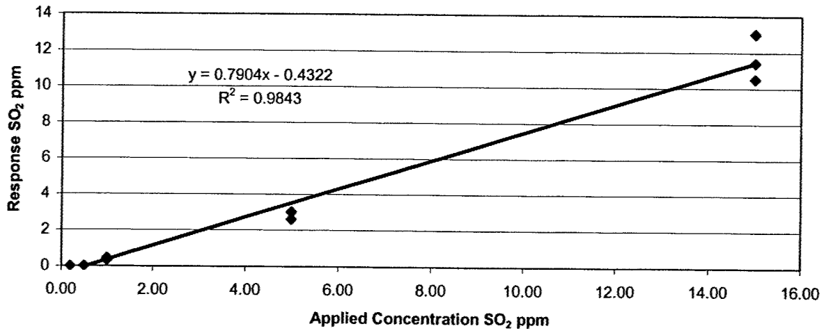
Dräger SO 2
