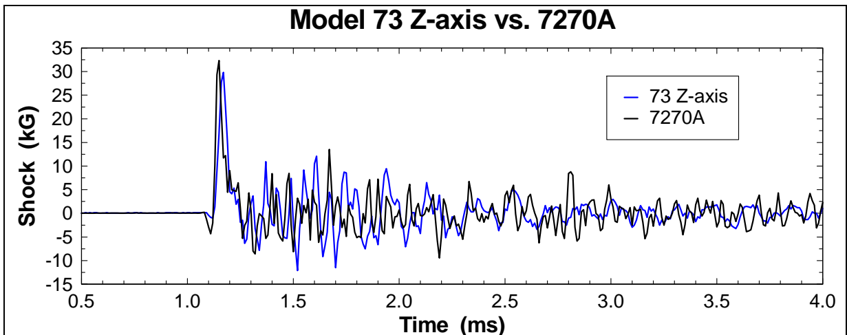
Figure 26. Test 6 of the triaxial accelerometer and Stycast epoxy (z axis).
