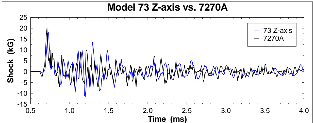
Figure 20. Test 3 of the triaxial accelerometer and Stycast epoxy (z axis).
