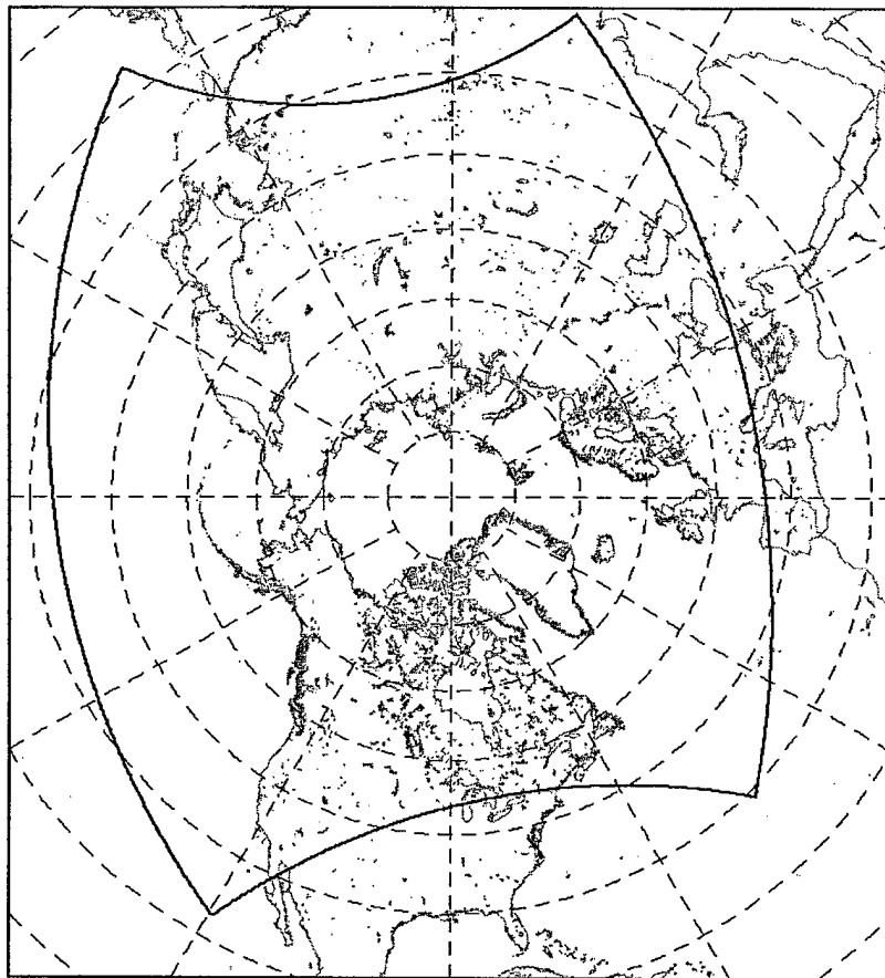
FIG. 1. Spatial domain of PIPS. The latitude spacing is 10^\circ and the longitude spacing is 30^\circ .
