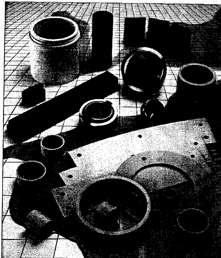
Tenmat Feroform
