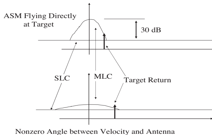
Fig. 6 — Doppler spectra
