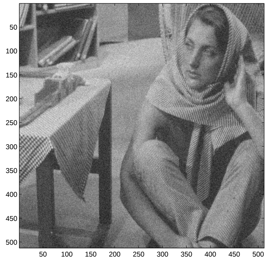
(q) Noisy
