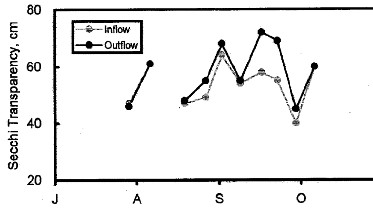
a. Secchi transparency
