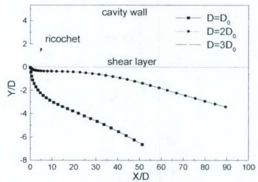
b) Trajectories of CG
