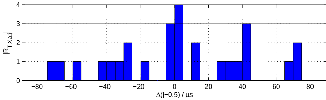
(d) Cross-correlation histogram |R_{T,X,\Delta,j}| using \Delta = 5
