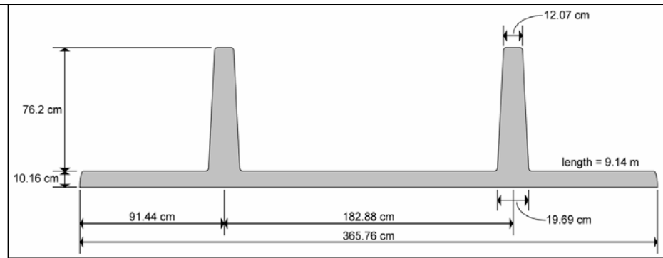
a. Dimensions
