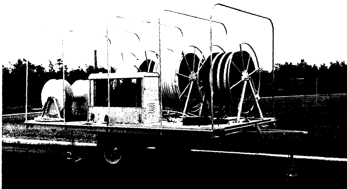
Fig. 2.1—Caisson trailer.
