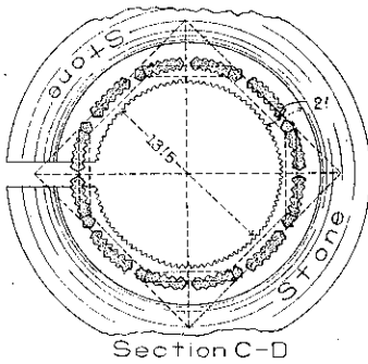
Section C-D
