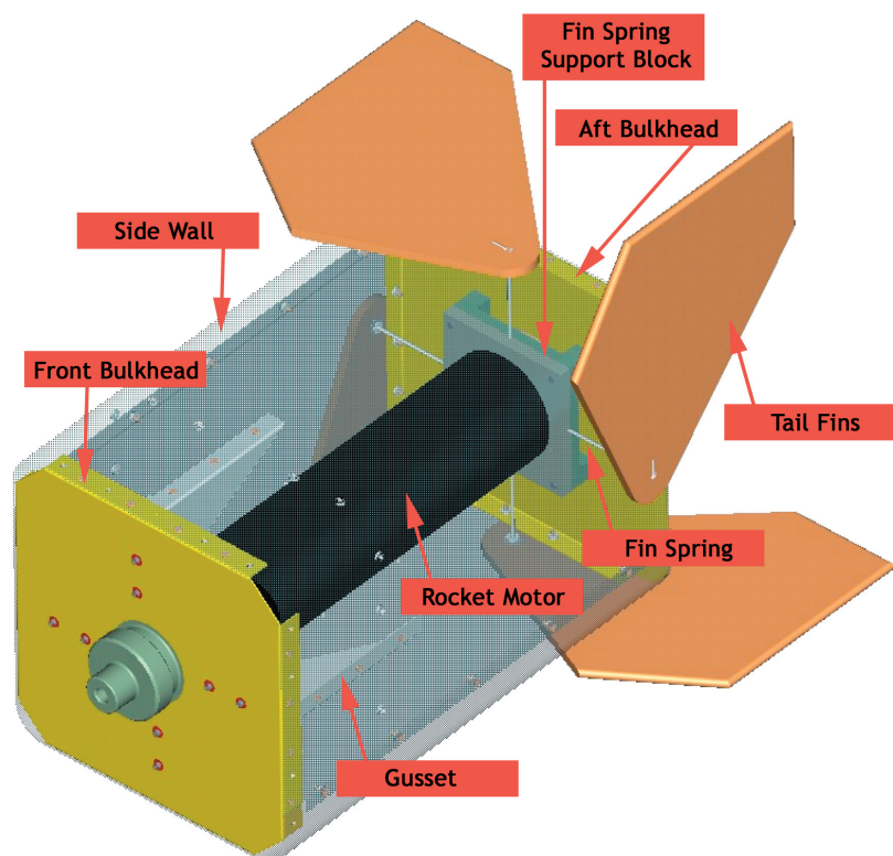
Fig. 16 — Aft subassembly
