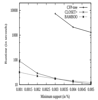
Fig. 21. Runtime comparison( T10I4D100K ).
