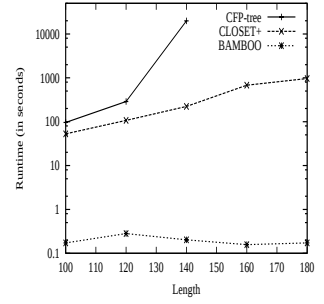
Fig. 19. Runtime comparison( gazelle ).
