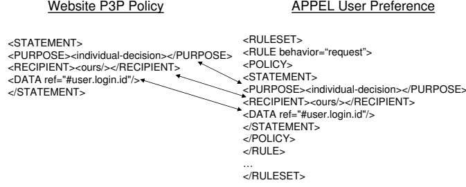
Fig. 1. P3P-APPEL matching
