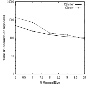
Fig. 7. Runtime ( pumsb* ).
