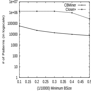
Fig. 4. # Patt. ( big-market ).
