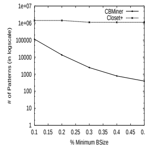
Fig. 2. # Patt. ( gazelle ).
