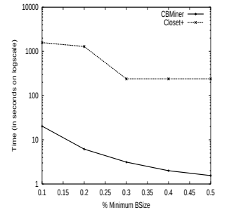
Fig. 3. Runtime ( gazelle ).
