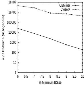
Fig. 6. # Patt. ( pumsb* ).
