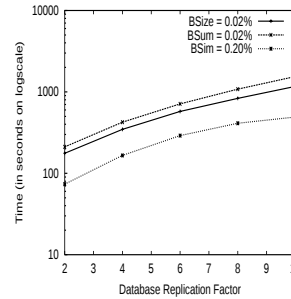
Fig. 18. scalability ( T20I10D100Kx ).
