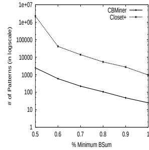
Fig. 10. # Patt. ( sports ).
