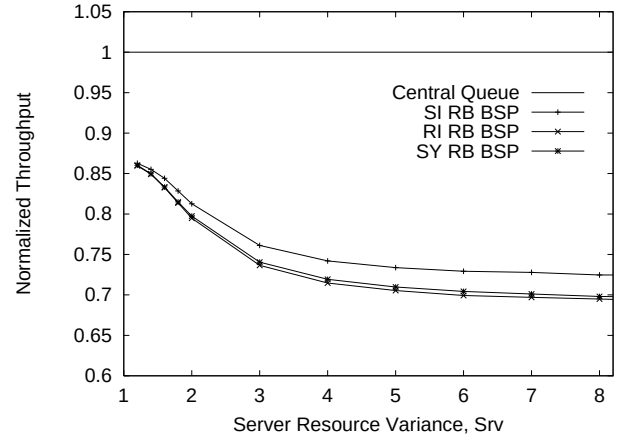
(d) Server Resource Correlation: Src=0.15
