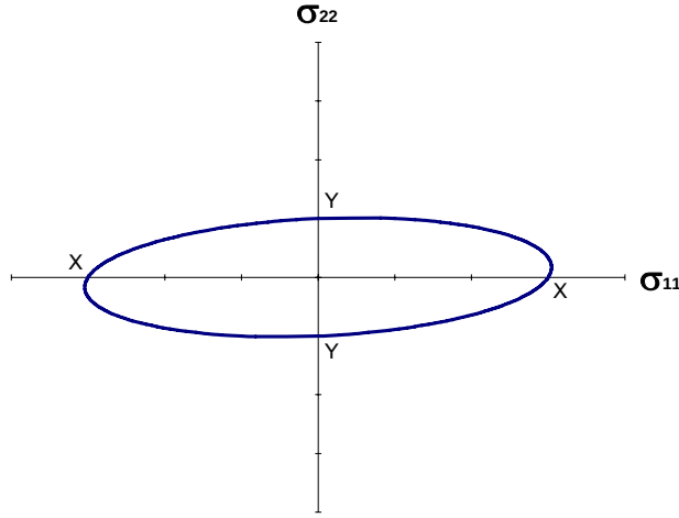
Fig. 7.5.3, Tsai Hill
