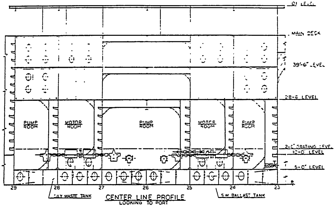
T-AO TWIN-SKEG
