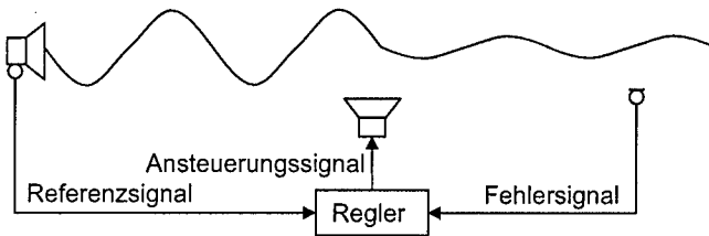
Abb. 1.4: Prinzipskizze zur Vorwärtsführung
