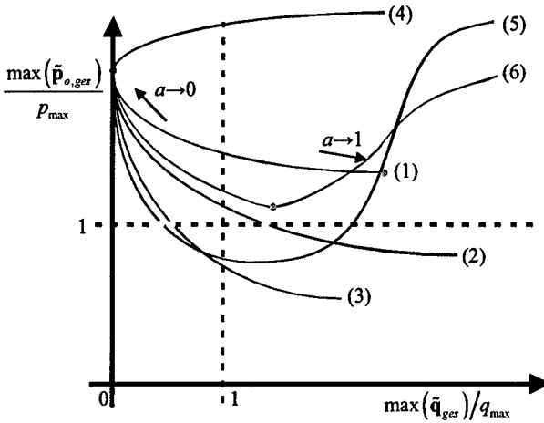
Abb. 4.1: Idealisierte p-q-Kurven
