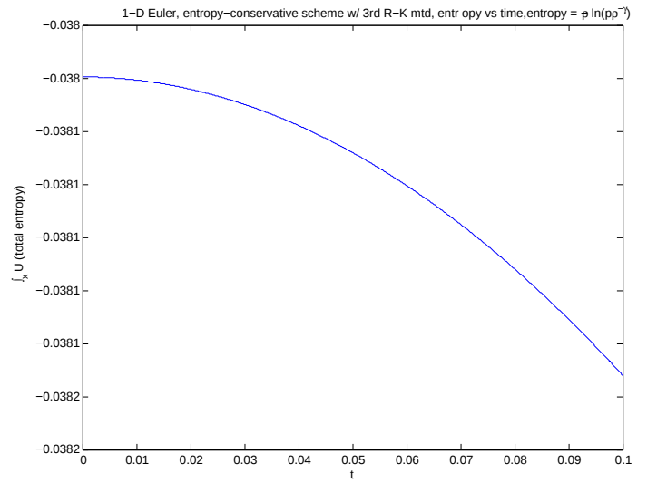
(d) Total entropy v.s. time
