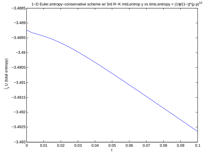
(d) Total entropy v.s. time
