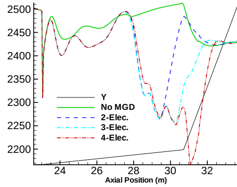
(d) u-Velocity(m/s)
