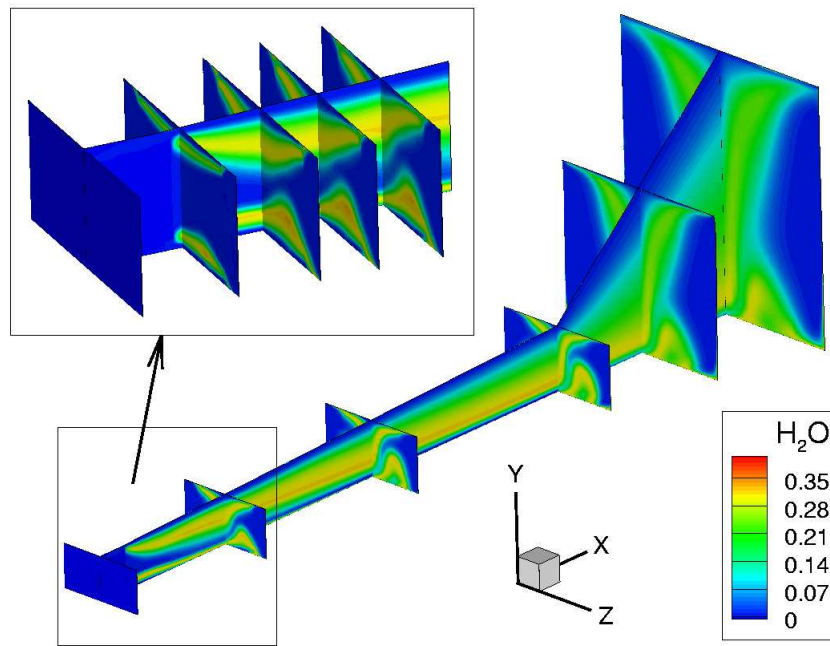
(b) Y_{H_2O}
