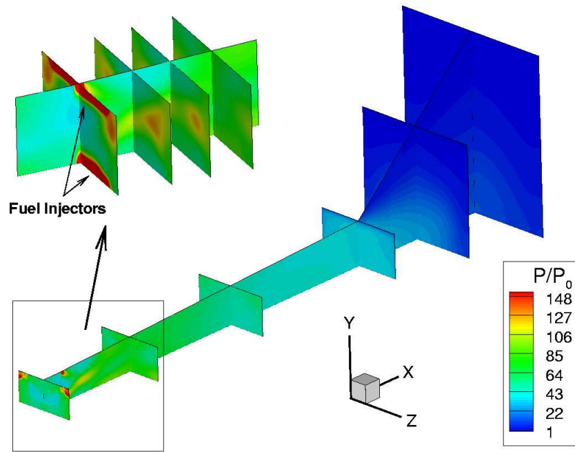
(a) P/P_0
