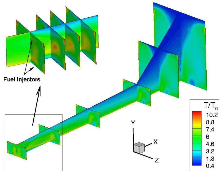
(b) T/T_0
