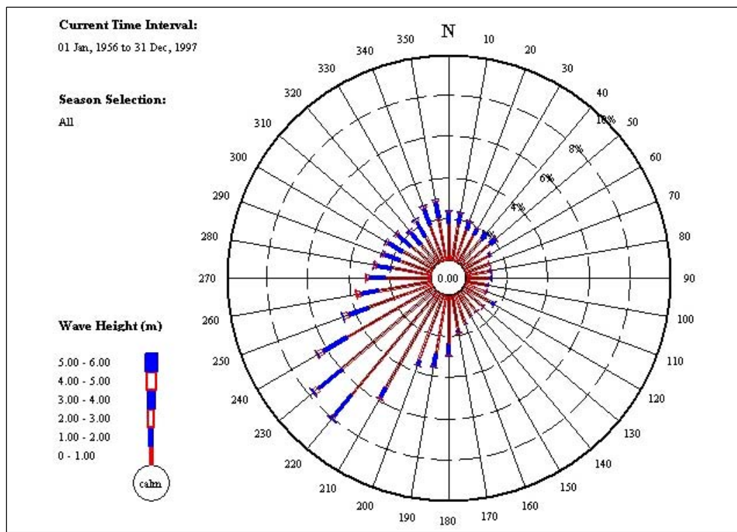
Figure B5. Wave height rose, Charlevoix, MI.
