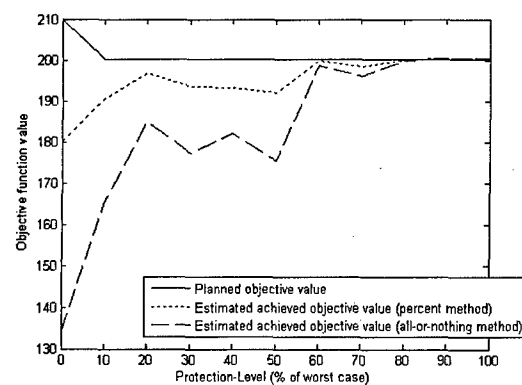
(d) Bertsimas/Sim Achieved Obj. Func.
