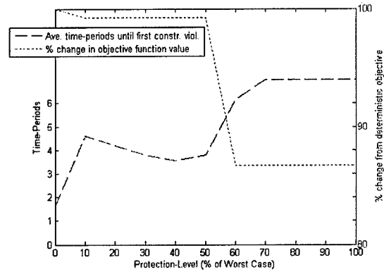
(d) Mean Time Until Failure
