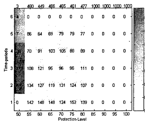
(d) Normal Hazard Rate Plot
