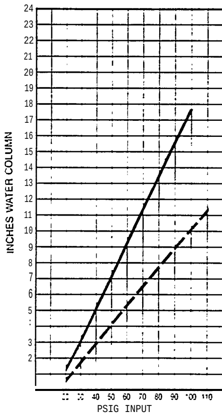
912/952 Transvector
