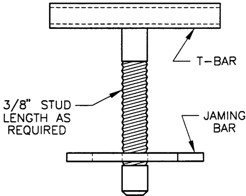
T-BAR ASSEMBLY
