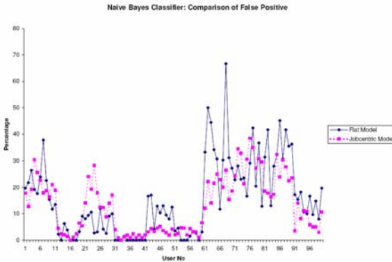
(d) Naive Bayes Model - False Positive Rate
