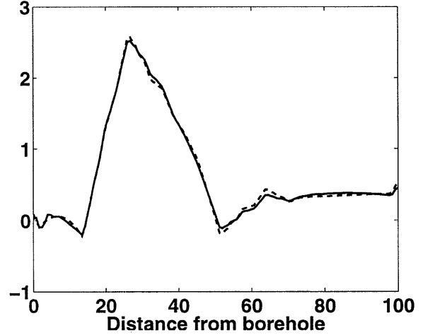
(d) \hat{g} (solid line) vs \hat{g}_{0.50} (dashed line)
