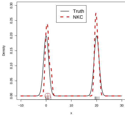
(d) NKC
