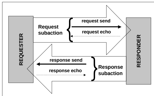
Fig. 1. SCI subactions.
