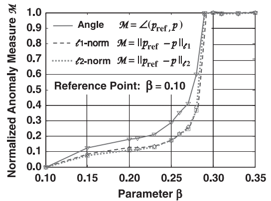
Fig. 5. Anomaly measure versus parameter \beta .
