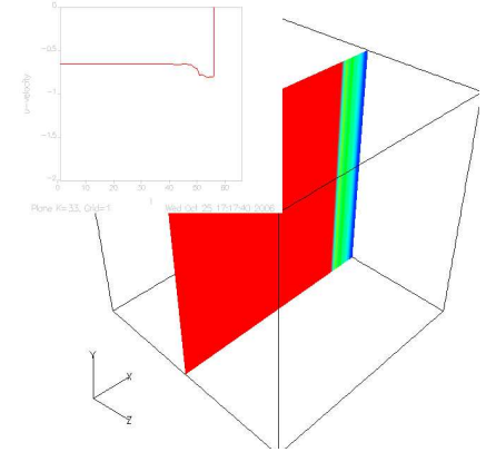
(d) Pressure wave t = t3 .
