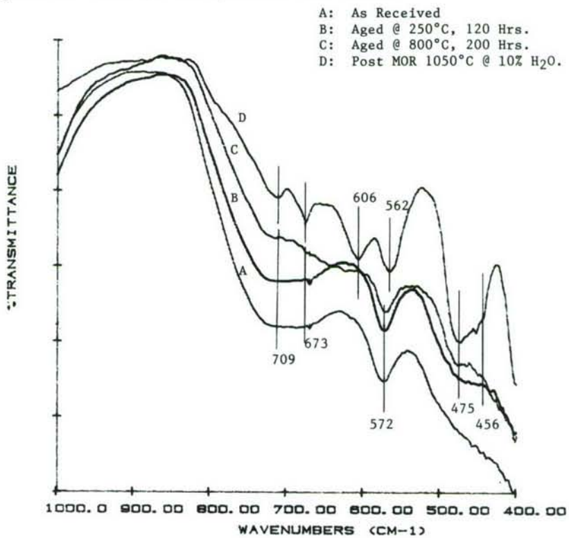
Figure 10. ATR FT-IR spectra for MS-PSZ.
