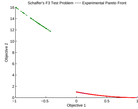
(d) Experimental Pareto Front
