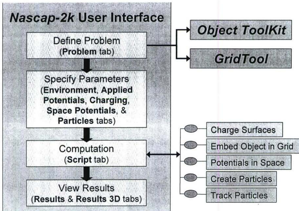
Figure 2. Nascap-2k Module Diagram.
