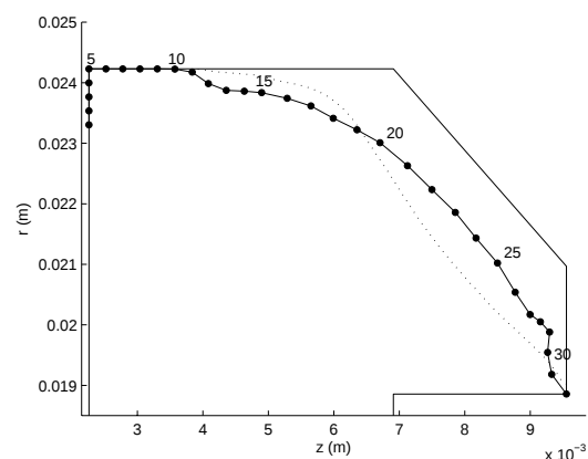
(d) Inner insulator, 932 hours.
