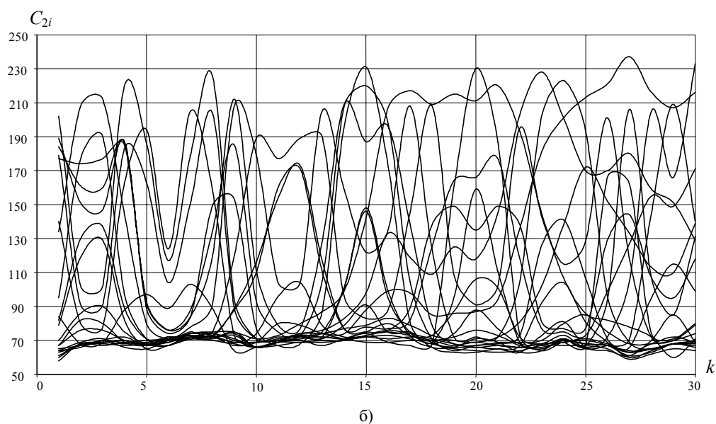
Рисунок 1 – Зависимости кодов от номера пакета (периода) при отсутствии ( C_{1i}(k) ) и наличии ( C_{2i}(k) ) срывных и помпажных явлений для группы контролируемых лопаток ( i=1, 2, \dots, 21 , ступень 5, замеры 31, 32).
