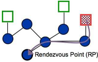
Fig. 4. A PIM Register message
