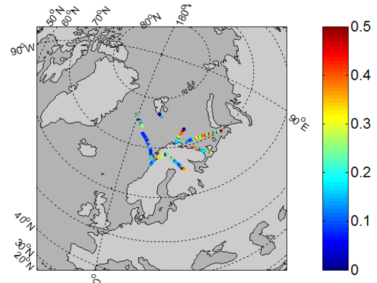
Sigma phi 8-11-2004-2 UT
