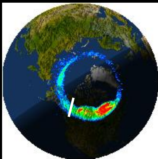
Polar UVI
