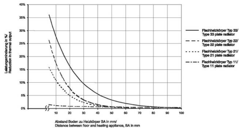
Bild B4. Leistungsminderung in Abhängigkeit vom Bodenabstand des Heizkörpers
