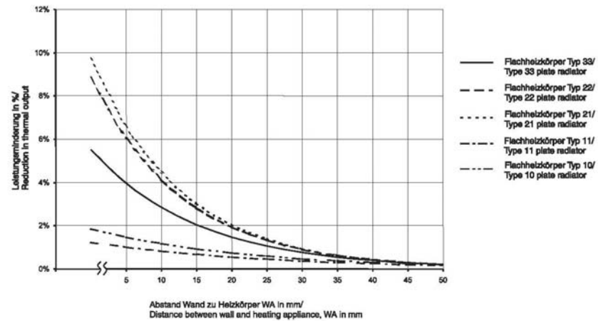
Bild B3. Leistungsminderung in Abhängigkeit vom Wandabstand des Heizkörpers
