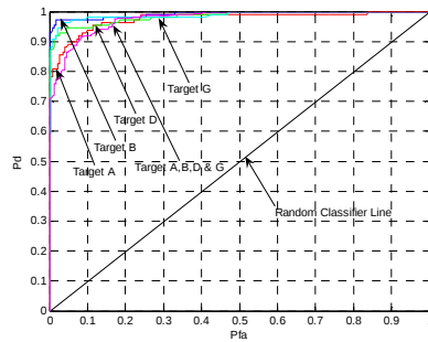
e) SOM features using HH, HV and VV
