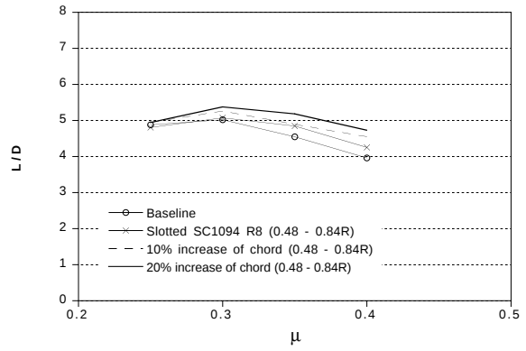
(d) Lift-to-drag ratio at C_T/\sigma = 0.12
