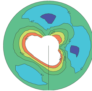
(b) \mu=0.15
