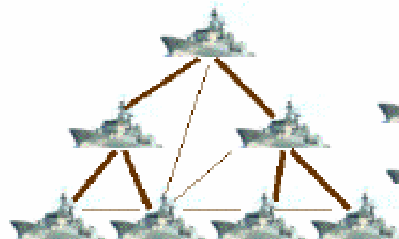
(b) Hierarchical
