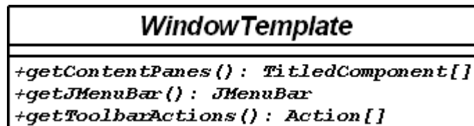
Figure 25 dsto.nef.core.swingui.WindowTemplate
