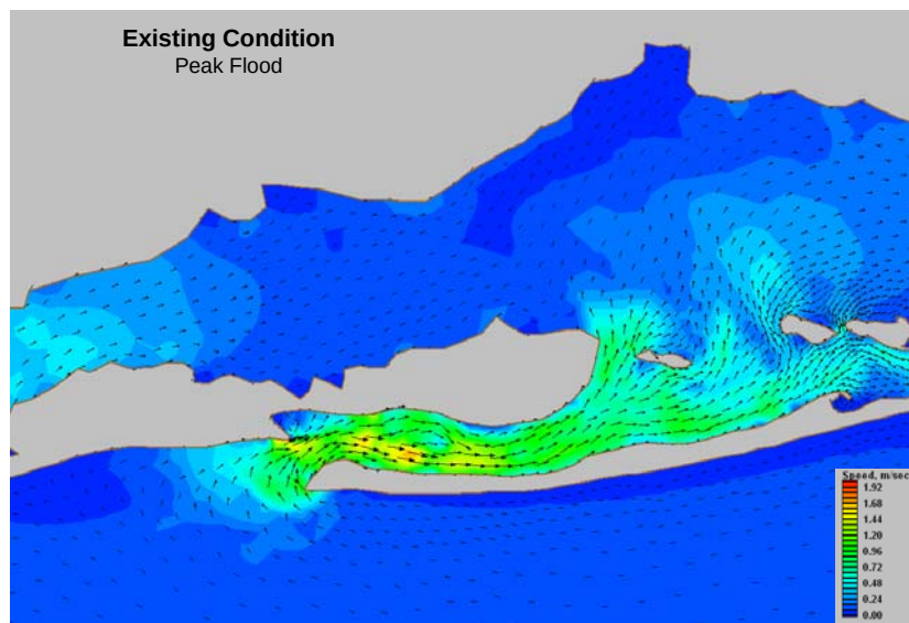
Fig. 4a. Existing inlet
