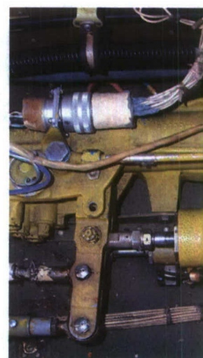
Rudder Actuator EA-6B
