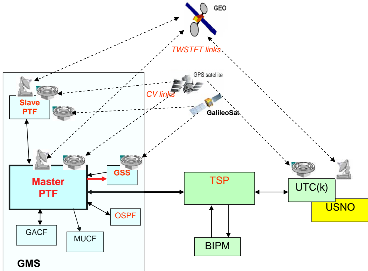
Fig. 2. The PTF Galileo/GPS scenario.
