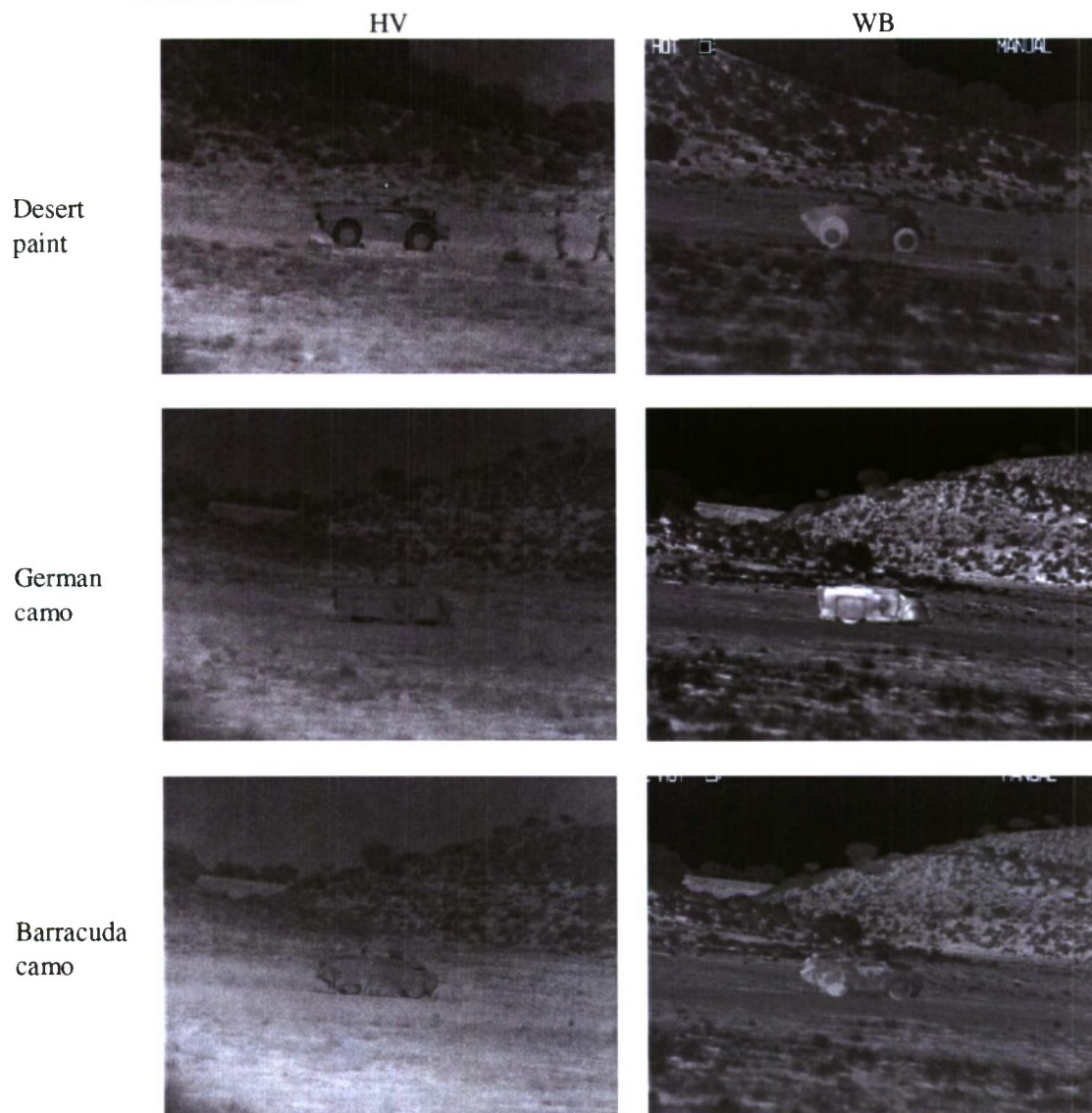
Figuur A.44 Digitale HV (linker kolom) en Lion Advance warmtebeeld (rechter kolom) zij aanzicht opnamen van een Fennek in een desert paint uitvoering (bovenste rij), met een Duits MCS (middelste rij), en met een Barracuda MCS (onderste rij).
